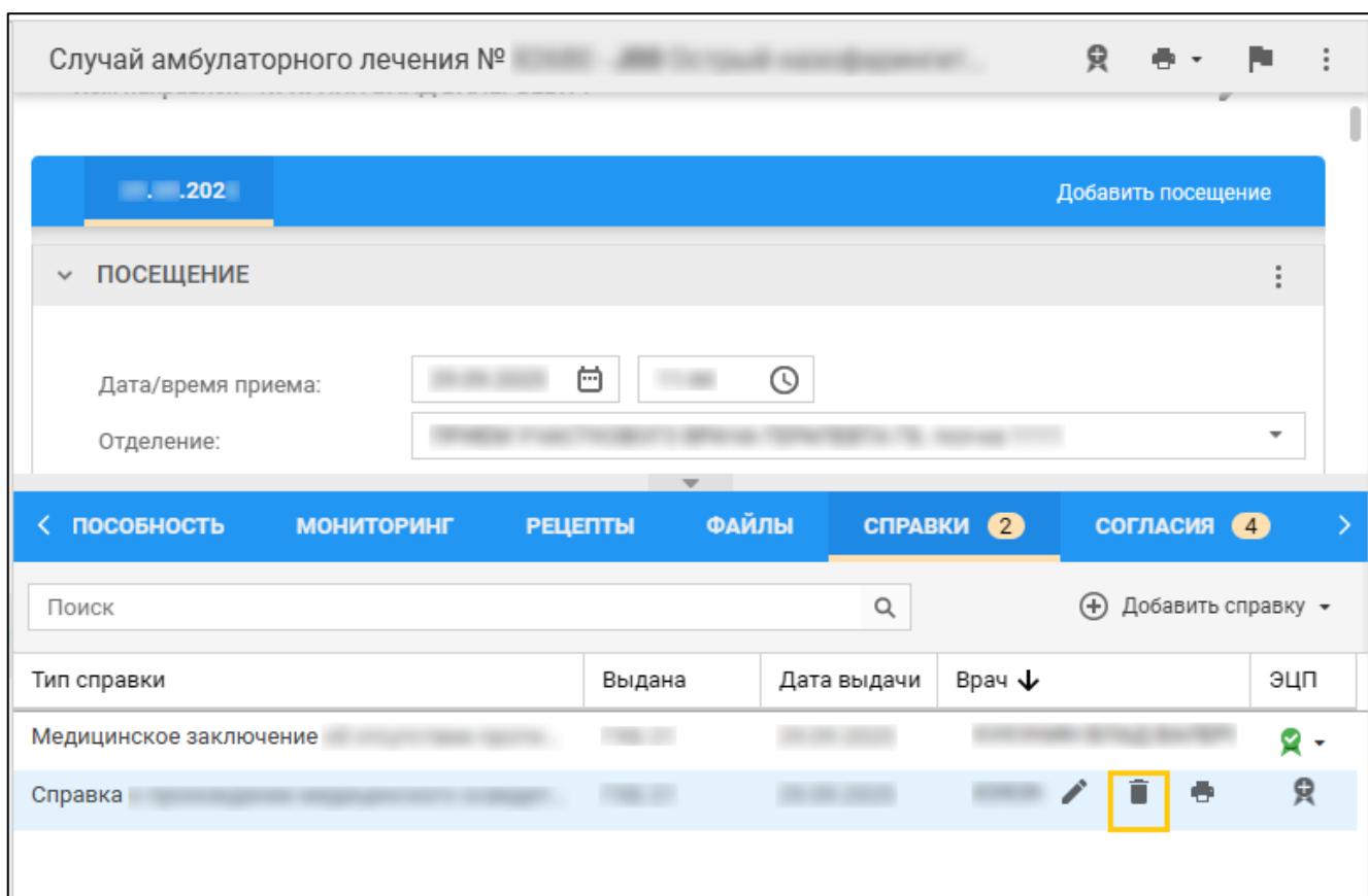
Рисунок 15 -- Удаление справки
